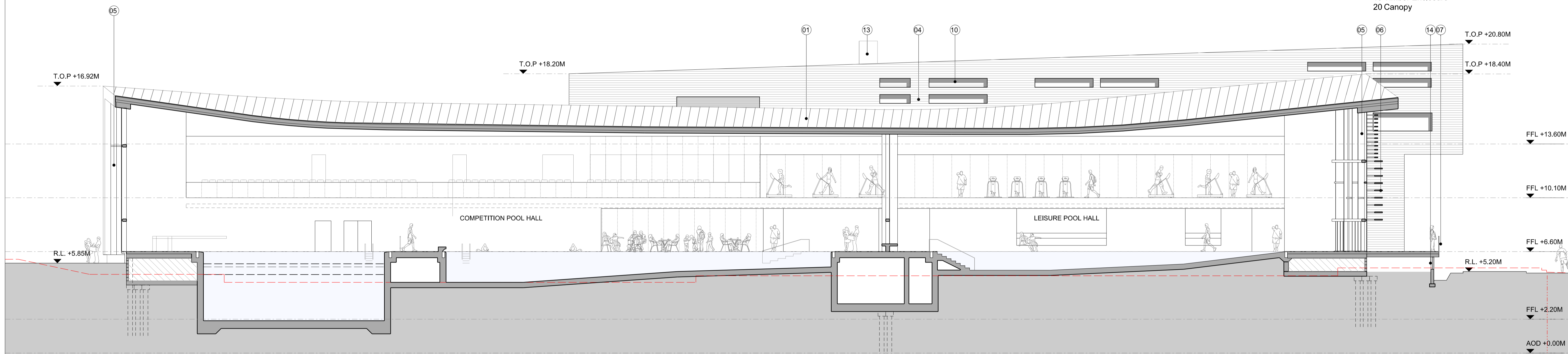
01 LONGITUDINAL SECTION D-D
